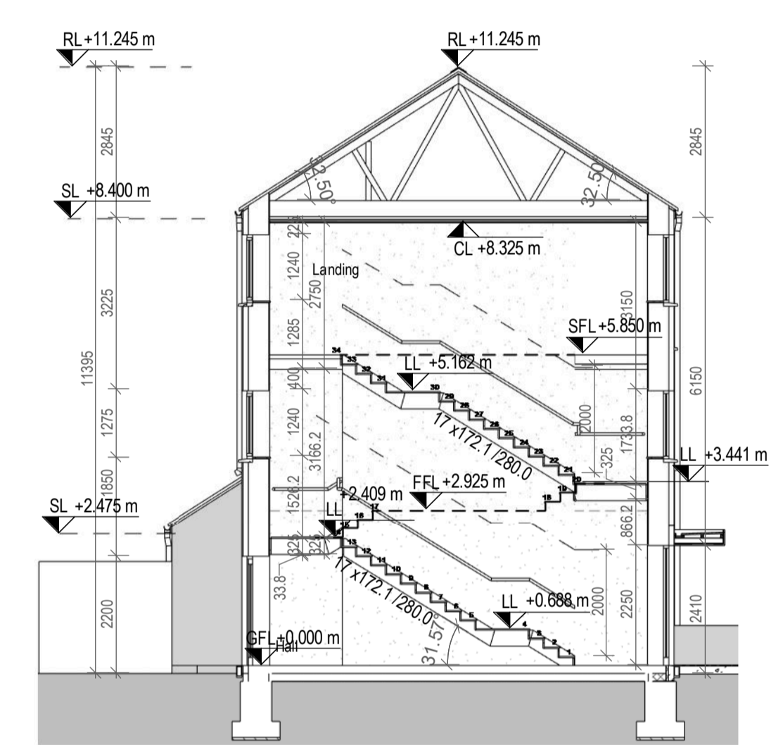
5 Section A-A 1 : 100
