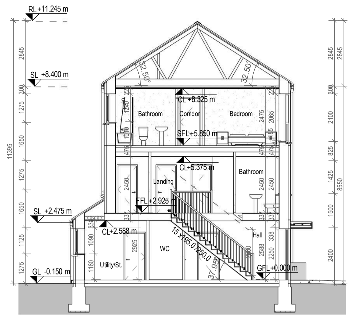
7 Section C-C 1 : 100
