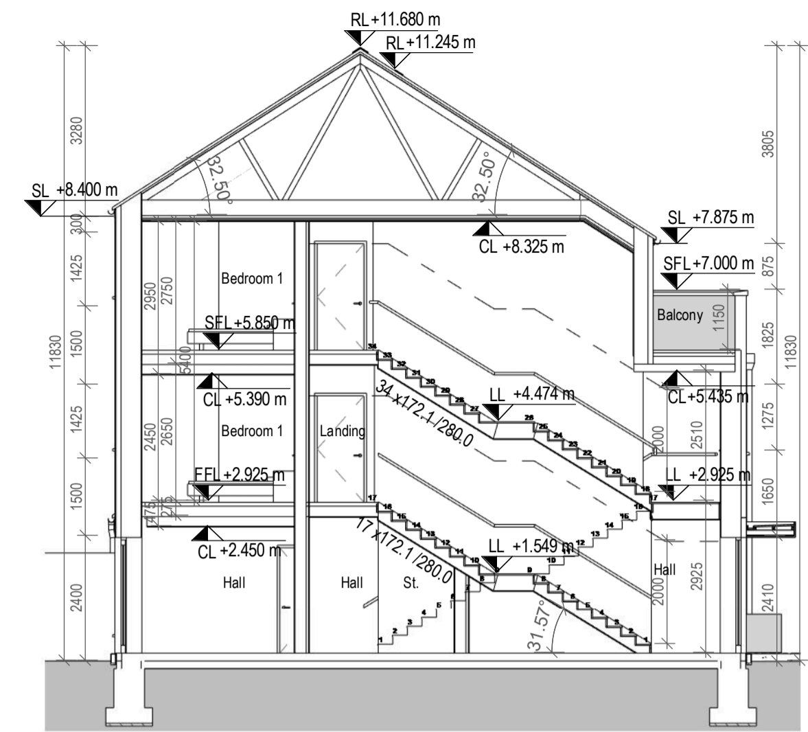
5 Section A-A 1 : 100
