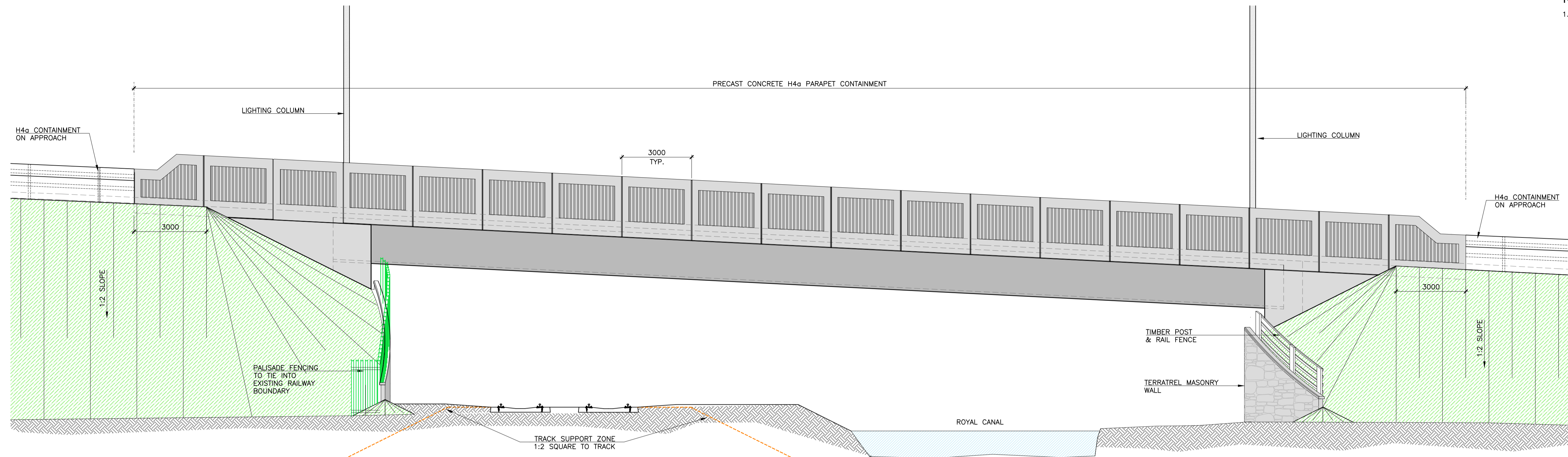
ELEVATION SCALE 1:100 A1 SCALE 1:200 A3
